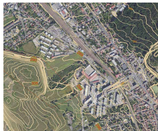
Prostorová studie s vrstevnicemi.
