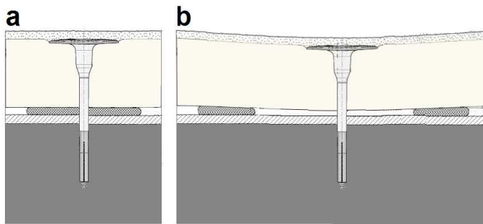
Obrázek 2 – a- správná poloha hmoždinky v místě lepícího tmelu, b – chybně umístěná hmoždinka (deska pruží případně se prohýbá)
