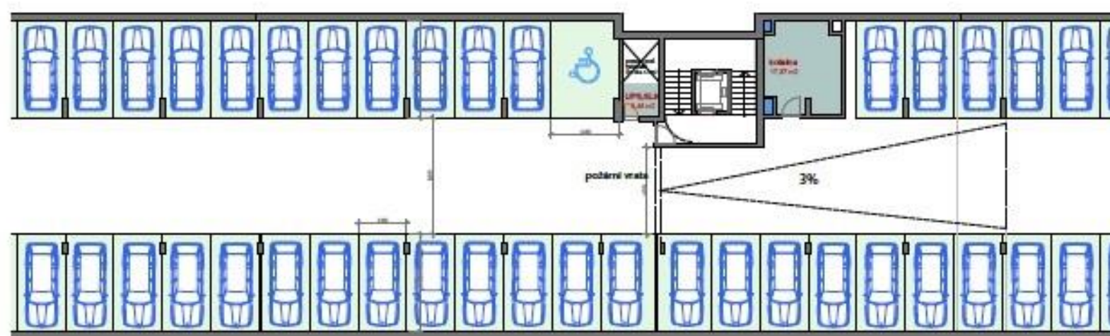
půdorys 1.PP
