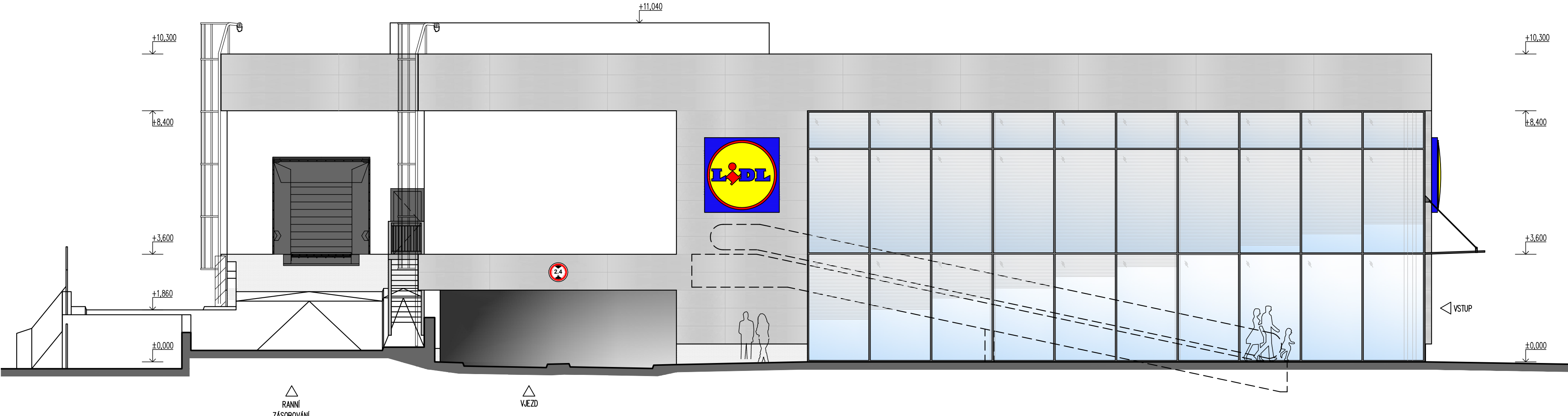
POHLED ZÁPADNÍ
